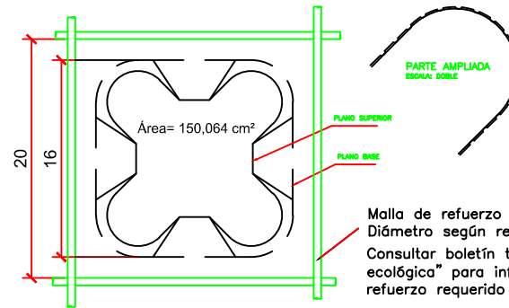
PLANO SIMPLE
