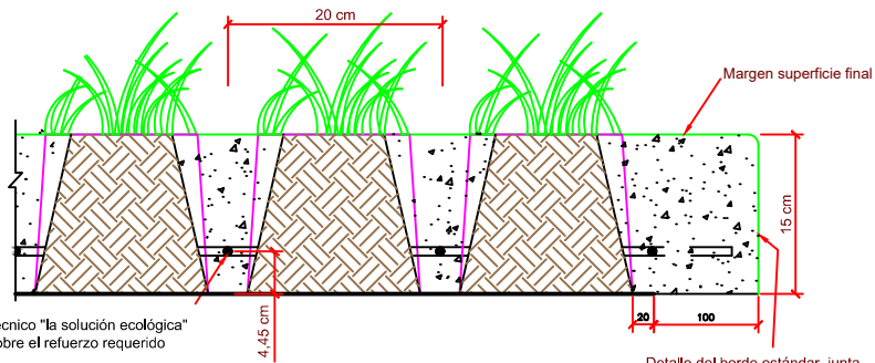
SECCIÓN - ALZADO
